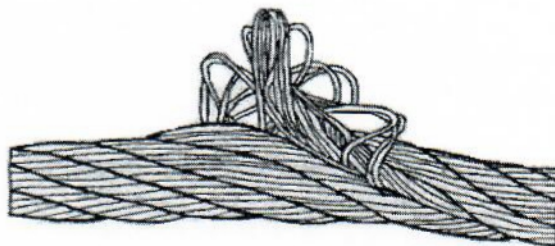
Рис. 11.4. Видавлювання металевго осердя
