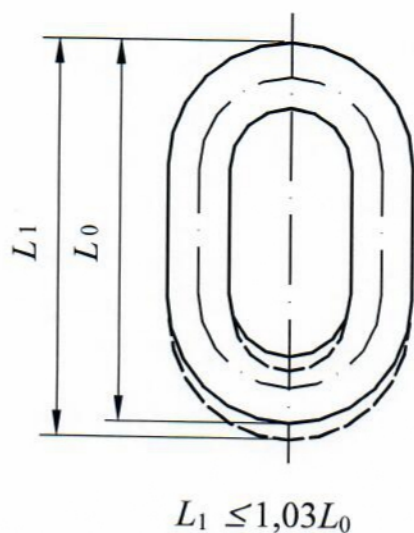
Рис. 12.1. Збільшення ланки ланцюга L_0 – первинна довжина ланки, мм; L_1 – збільшена довжина ланки, мм
