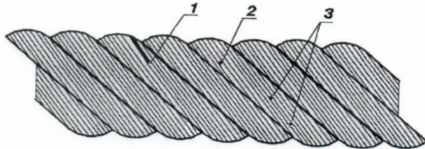
Рис. 11.1. Приклад визначення кількості обривів зовнішніх дротів сталевого каната
