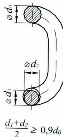
Рис. 12.2. Зменшення діаметра перерізу ланки ланцюга d_0 – первинний діаметр, мм; d_1, d_2 – фактичні діаметри перерізу ланки, виміряні у взаємно перпендикулярних напрямках, мм
